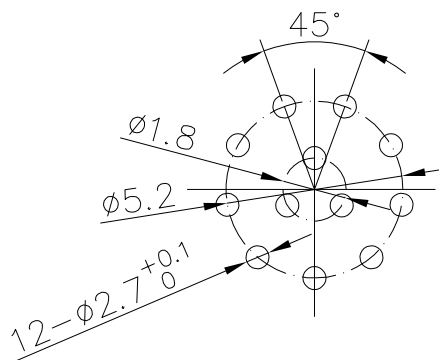
PCB dimensions
