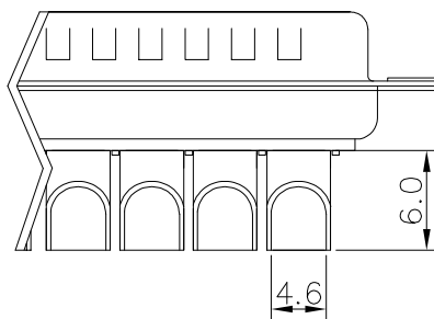
40A
