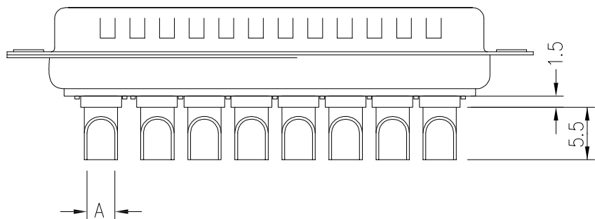
10A,20A,30A
