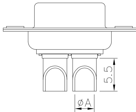
10A,20A,30A
