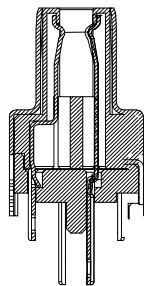
A-A section
