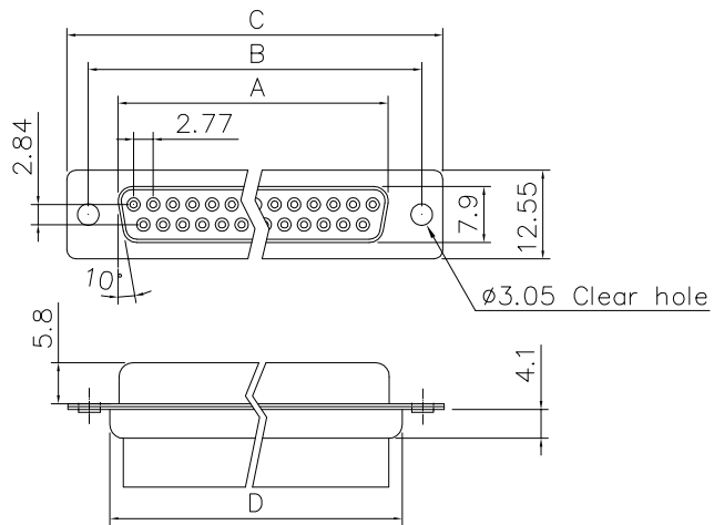
9,15,25,37pin
