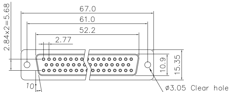
9,15,25,37pin
