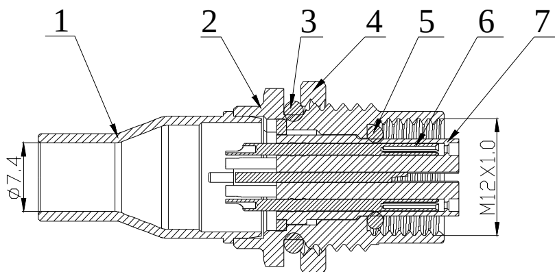
截面 A-A
