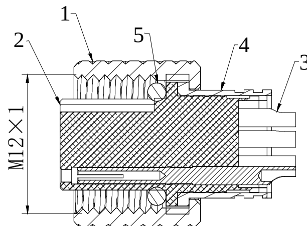
截面 A-A
