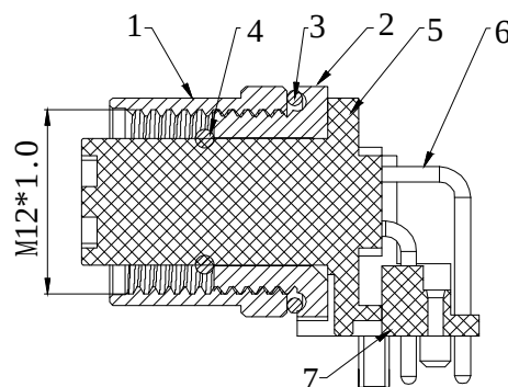
截面 A-A
