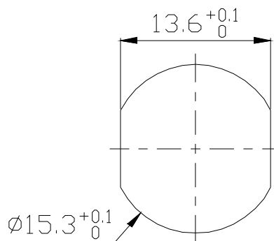
面板开孔尺寸
