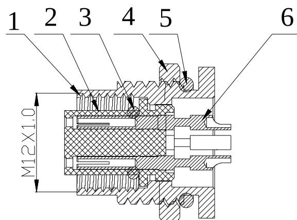
截面 A-A
