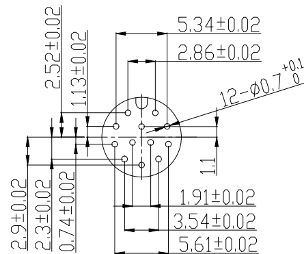
开板尺寸
