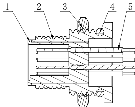
截面A-A
