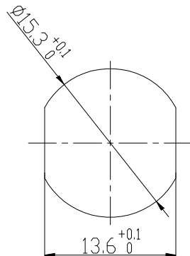
开板尺寸
