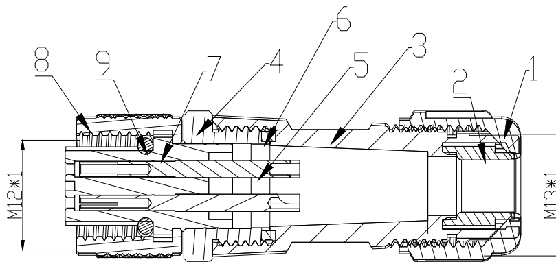
截面A-A
