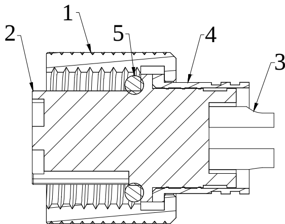
截面 A-A
