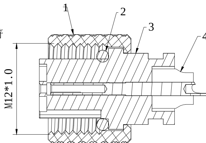
截面 A-A
