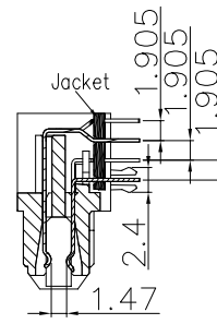
A-A section
