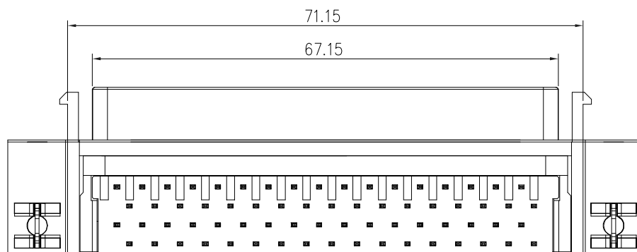
PCB EDGE
