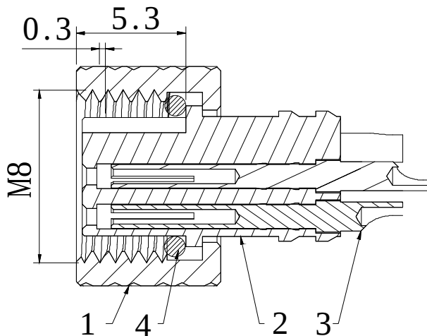
截面 A-A
