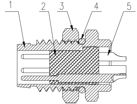
截面A-A
