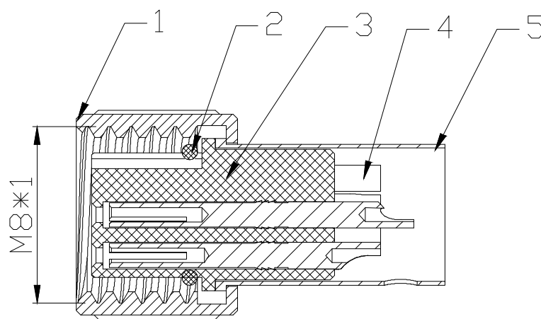
截面A-A
