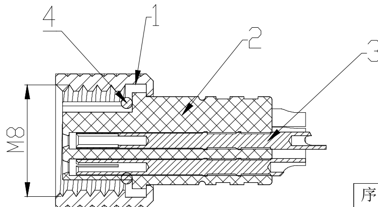
截面 A-A
