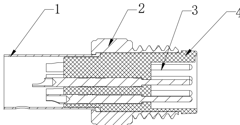
截面A-A
