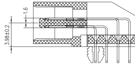
SECTION D-D SCALE 2:1
