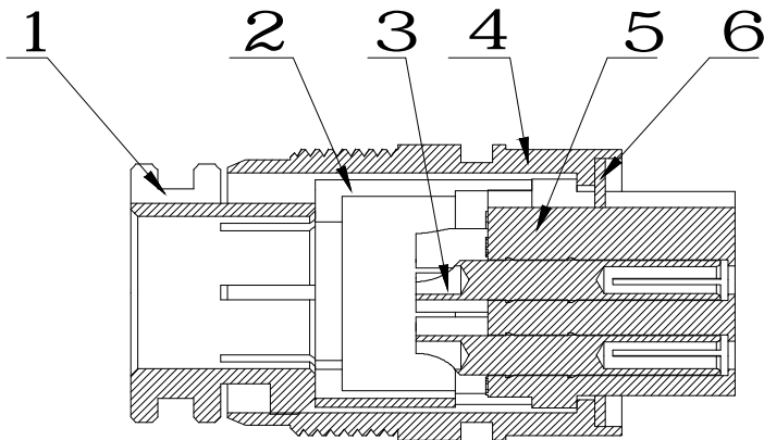
截面 A-A
