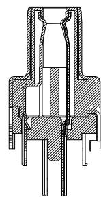
剖面 A-A
