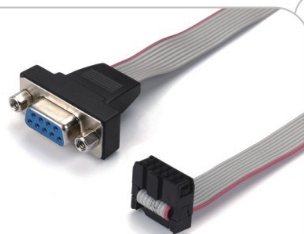
D-SUB 9P母头排线前铆螺母
